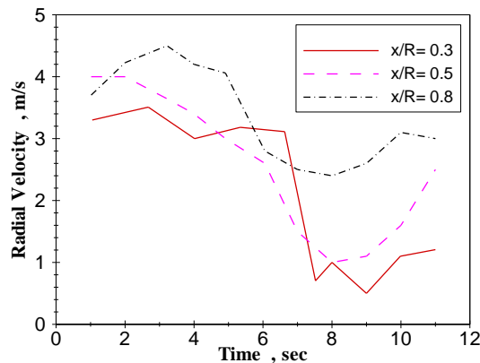
شکل ۱ - تغییرات سرعت شعاعی نسبت به زمان (B Nazanin ۱۰ pt, Bold)
